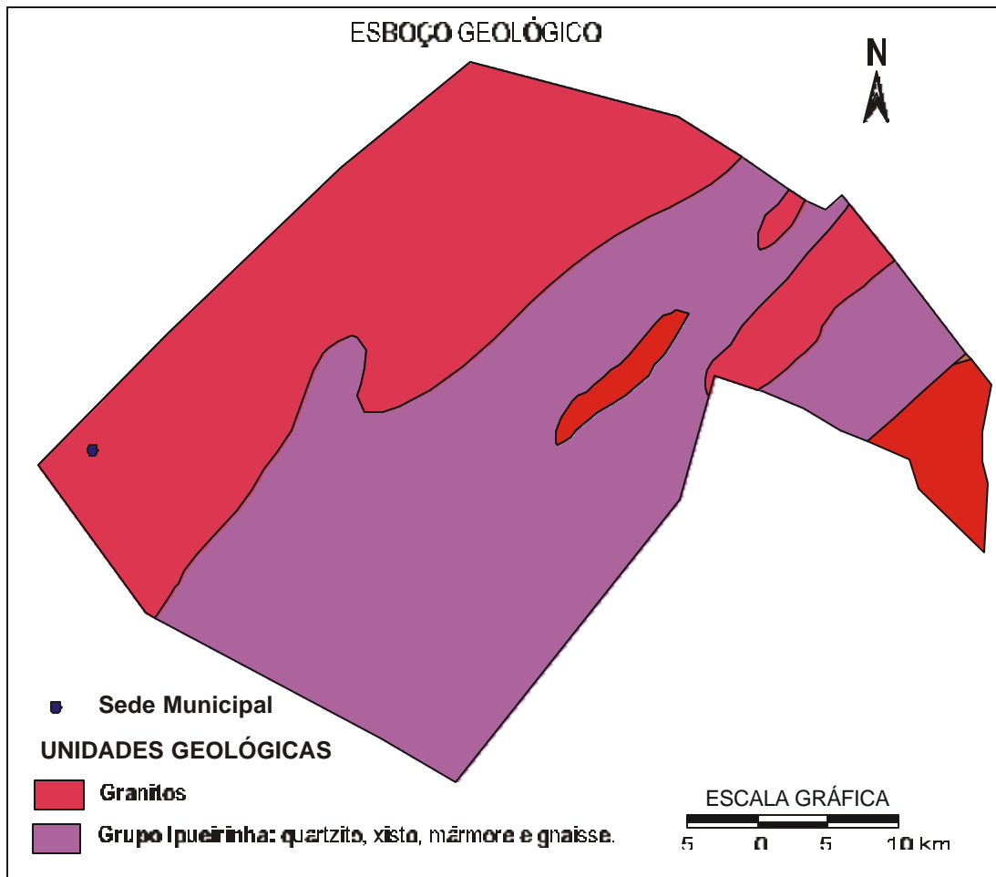
Figura 3– Esboço Geológico do Município de Caridade do Piauí.
