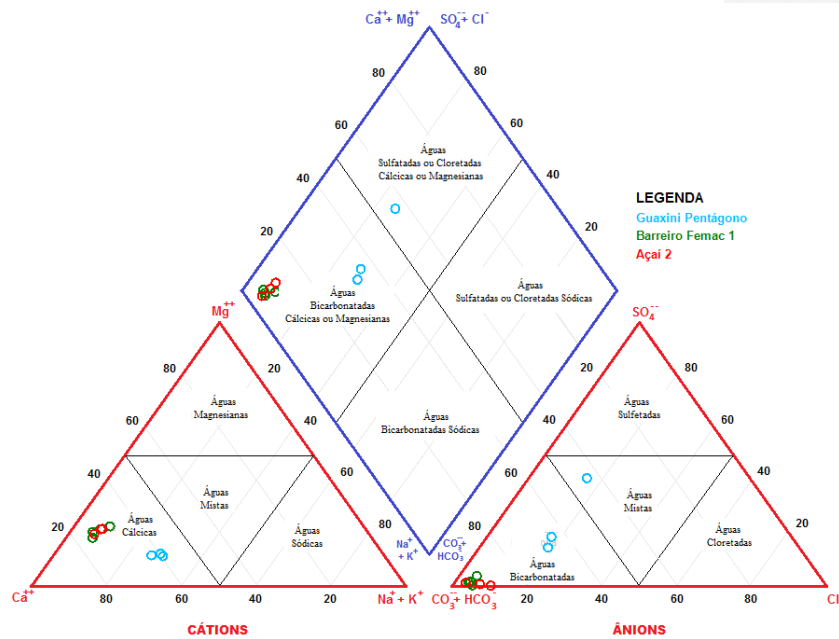
Figura 2 – Diagrama trilinear de Piper de amostras da água subterrânea. Período Seco. 1ª, 3ª e 4ª campanha de amostragem. Dezembro de 2016, 2017 e 2018. Classificação Iônica dos 03 poços RIMAS-BE (Salinópolis). Águas predominantemente Cálcica-Bicarbonatadas. Poço Guaxini Pentágono apresentou classificação Cálcica Mista em 2018.
